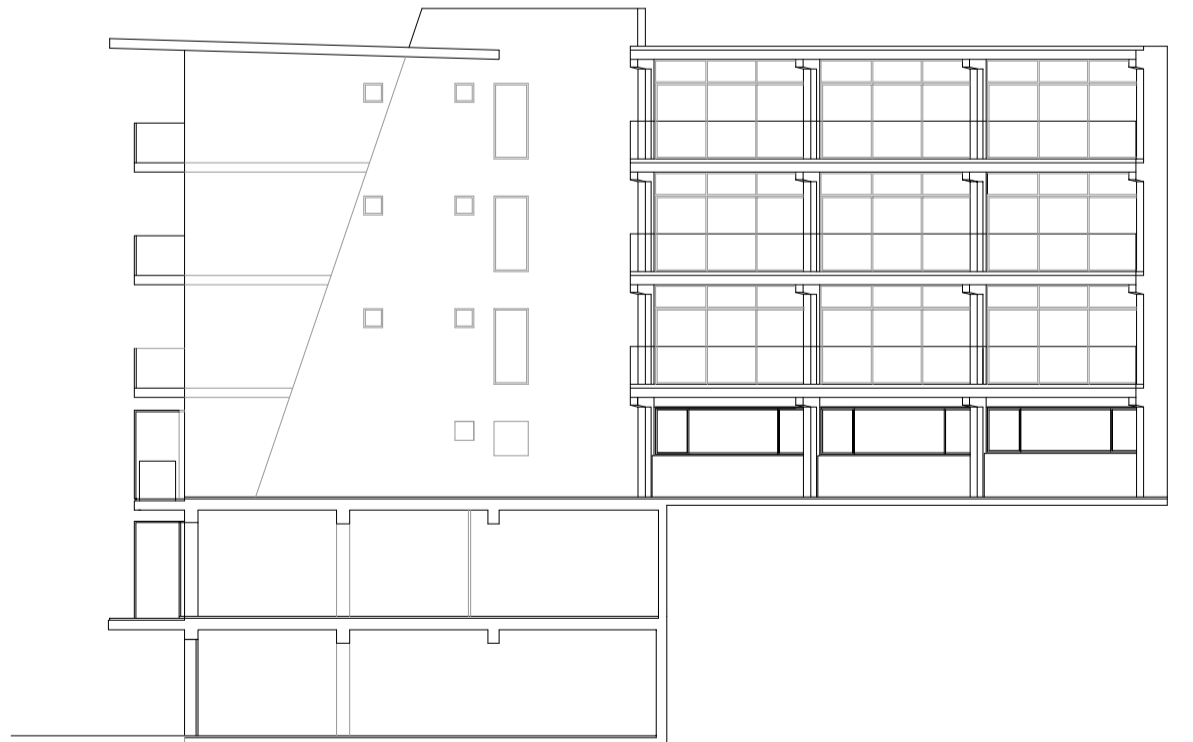
ALÇAT LATERAL
