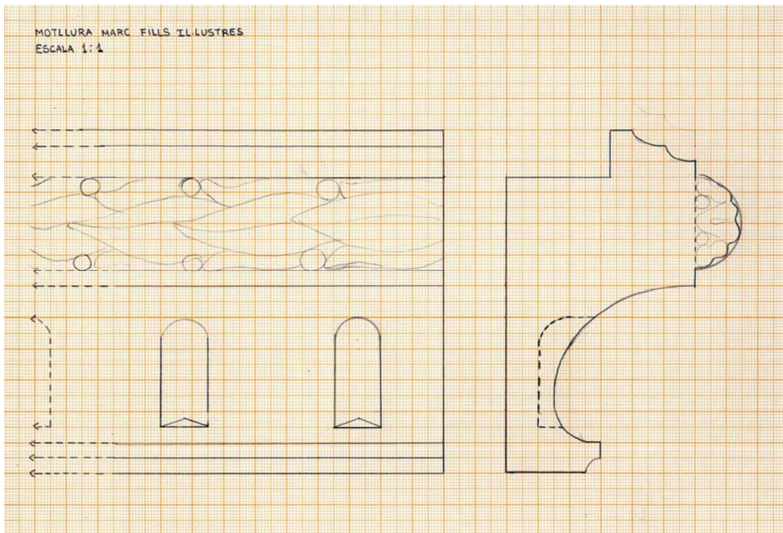
Croquis d'una secció de la vasa. Alçat i perfil de la motllura.
