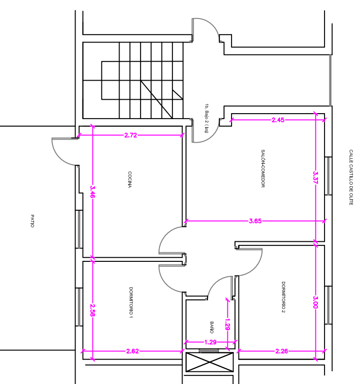
PLANTA BAJA 0 0,5 1,5 2,5 CALE ENTRE BLOQUES
