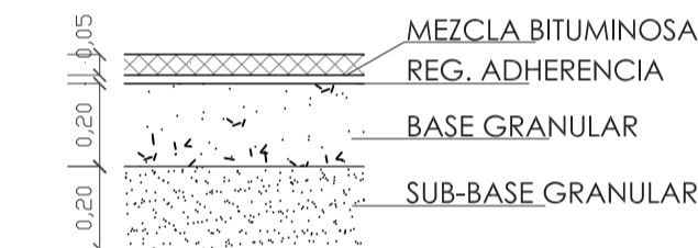
DETALLE PAVIMENTO E:1/20
