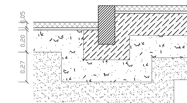
DETALLE PAVIMENTO E:1/20
